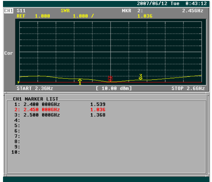
V.S.W.R
