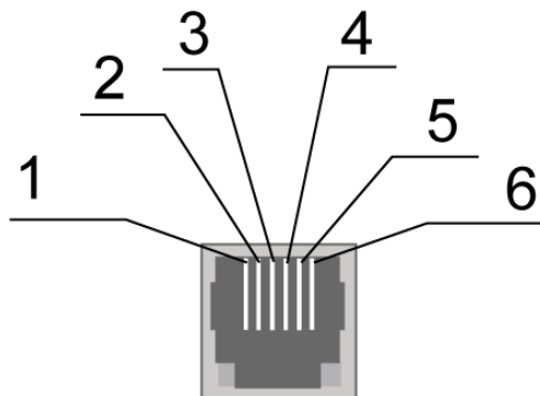
Рис. 2.4. Разъём питания
